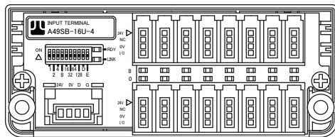
A49SB-16U-4
