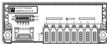
A. 出力用コネクタ (e-con 住友スリーエム 製)
