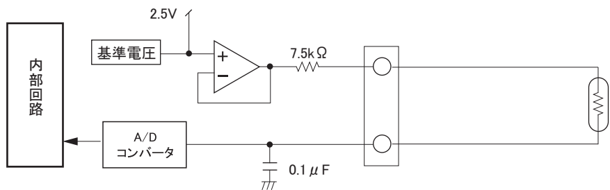
■サーミスタ入力回路特性
