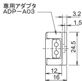
ADP-A03による取付図
