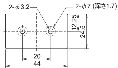
ADP-A03による取付図
