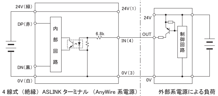
4 線式 (絶縁) ASLINK ターミナル (AnyWire 系電源)
