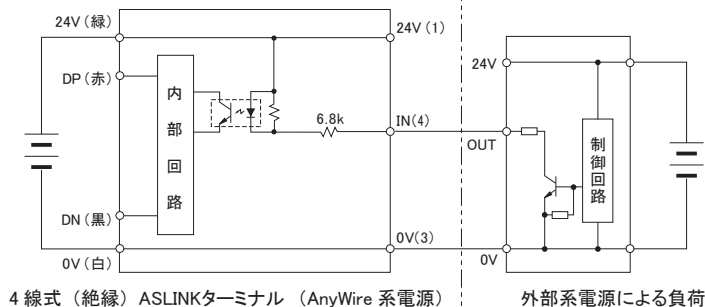
4線式(絶縁)ASLINKターミナル (AnyWire系電源)
