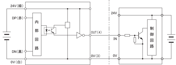
4 線式 (絶縁) ASLINK ターミナル (AnyWire 系電源)
