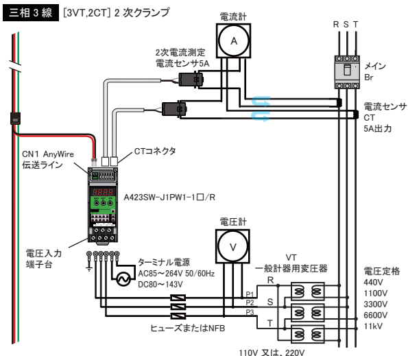
三相 3 線 [3VT,2CT] 2 次クランプ
