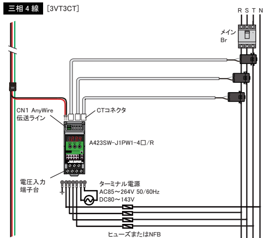
三相 4 線 [3VT3CT] 2 次クランプ
