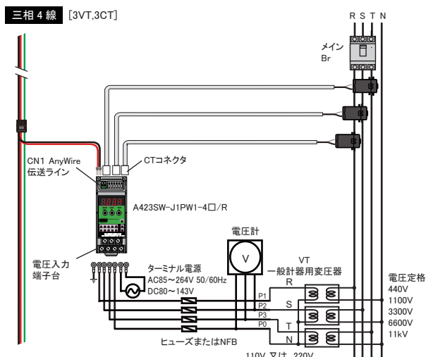
三相 4 線 [3VT,3CT] 2 次クランプ
