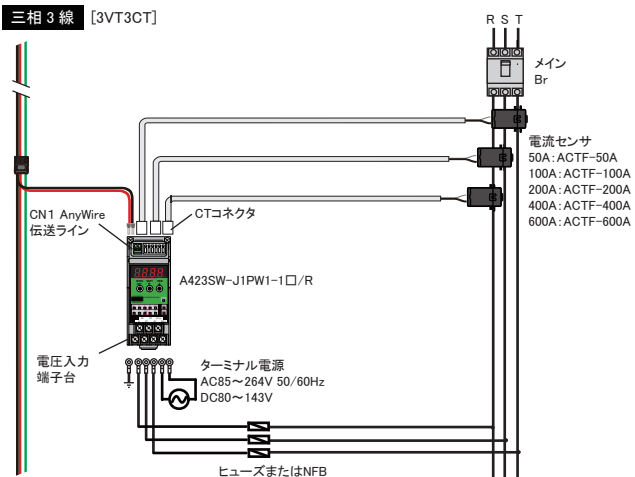
三相 3 線 [3VT3CT] 2 次クランプ
