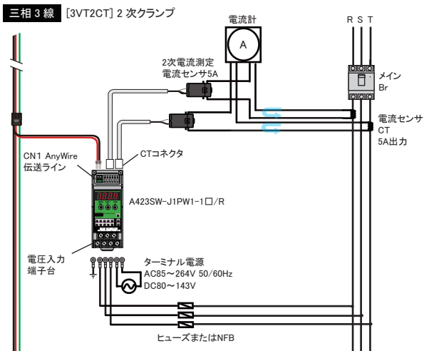
三相 3 線 [3VT.2CT]
