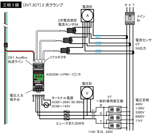
三相 3 線 [3VT,3CT] 2 次クランプ
