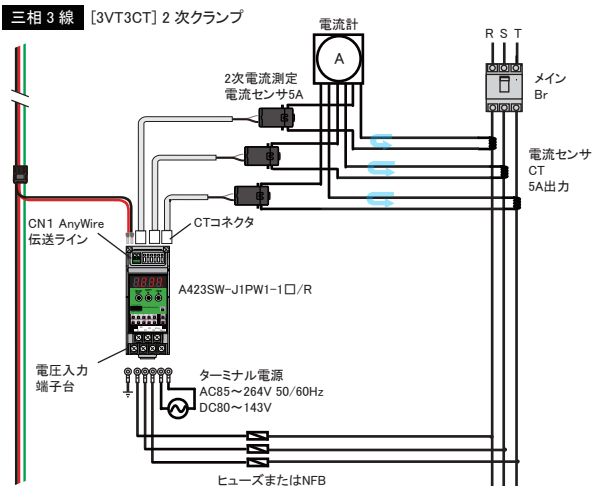
三相 3 線 [3VT,3CT]
