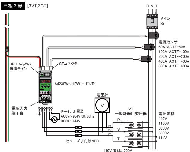
三相 3 線 [3VT,3CT] 2 次クランプ
