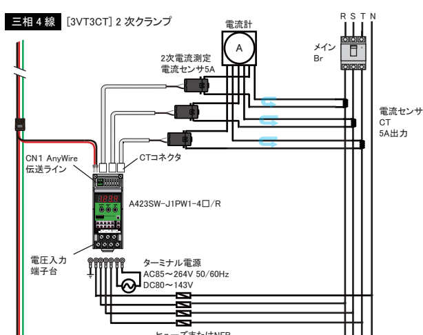
三相 4 線 [3VT,3CT]
