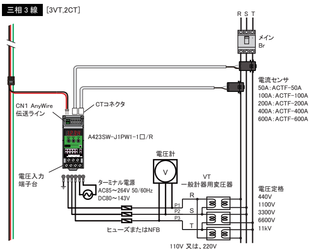
三相 3 線 [3VT,2CT] 2 次クランプ
