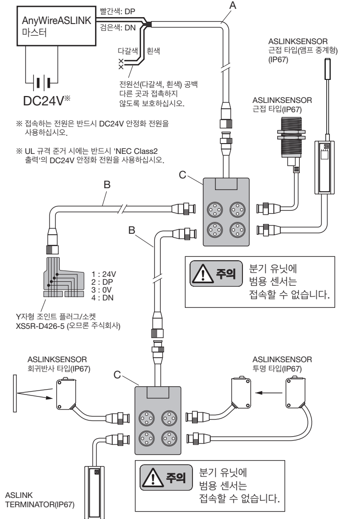
A 방수 간선 케이블(1.25mm²)
