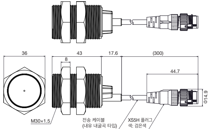
BS-K1117C-M30-3012
