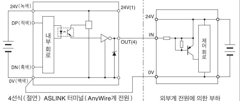
4선식 (절연) ASLINK 터미널 (AnyWire계 전원)
