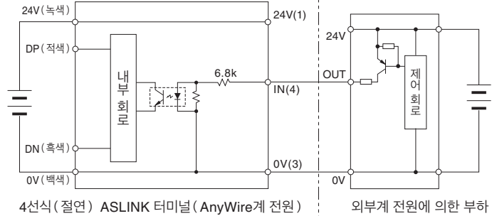
4선식(절연) ASLINK 터미널 (AnyWire계 전원)
