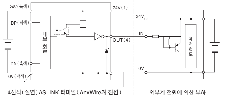
4선식 (절연) ASLINK 터미널 (AnyWire계 전원)
