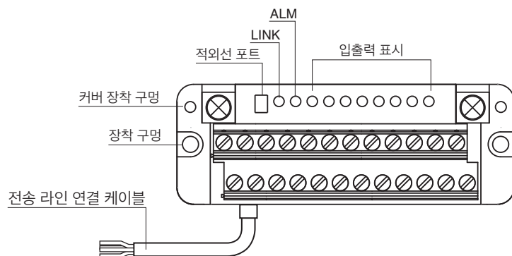
Euro 단자대
