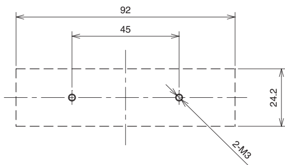
<ADP-T96D 장착 구멍 치수>
