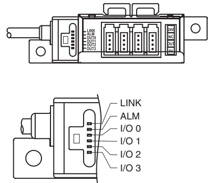
LED 표시부
