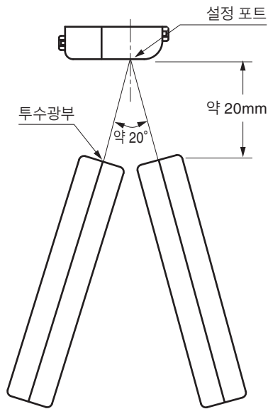
[윗면에서 본다]
