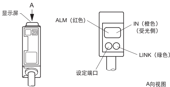
A向视图
