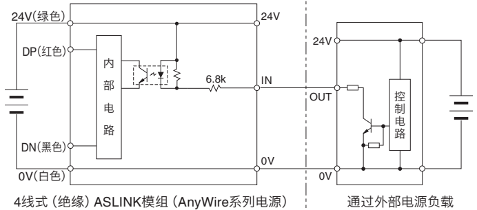
4线式 (绝缘) ASLINK模组 (AnyWire系列电源)
