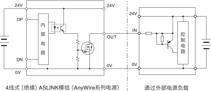
4线式 (绝缘) ASLINK模组 (AnyWire系列电源)
