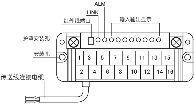
标准端子台
