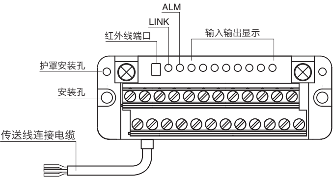
Euro端子台
