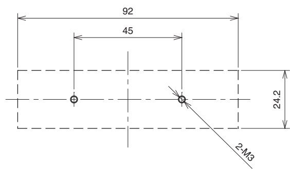
<ADP-T96D安装孔尺寸>
