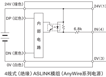
4线式 (绝缘) ASLINK模组 (AnyWire系列电源)
