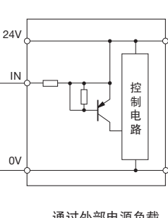
通过外部电源负载
