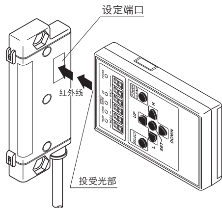
■遥控头连接状态的形象图
