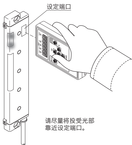
■操作形象图
