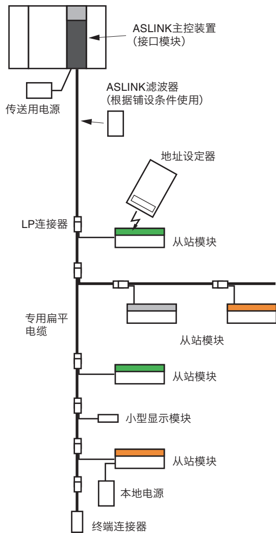
■配置示意图
